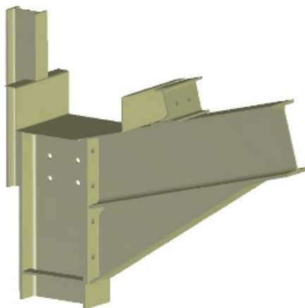
Noeud de charpente métallique réalisé avec des profil IPN.
