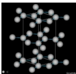
Graphite : structure hexagonale de paramètre a=0,246 nm et c=0,670 nm
