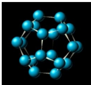
Le plus petit fullerène : C 20
