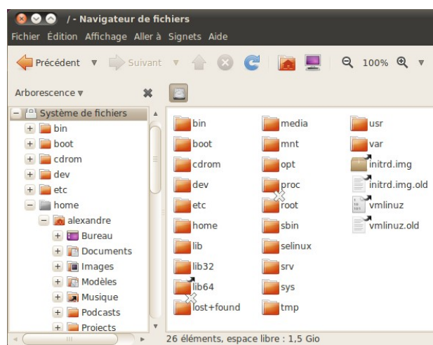
Arborescence Linux
