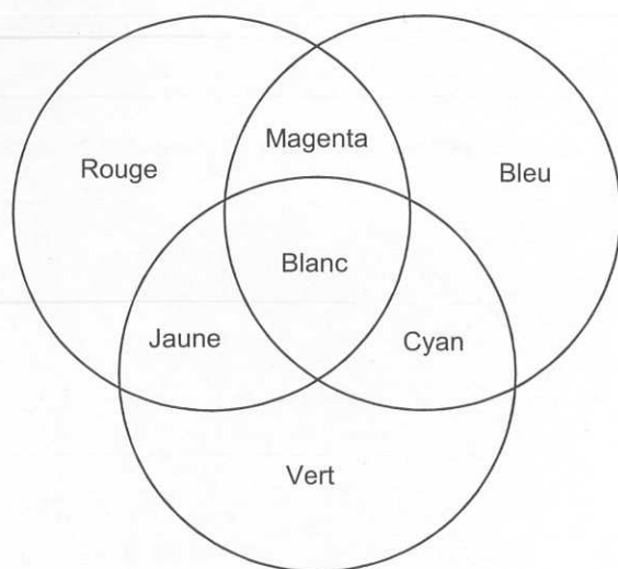
Synthèse additive
