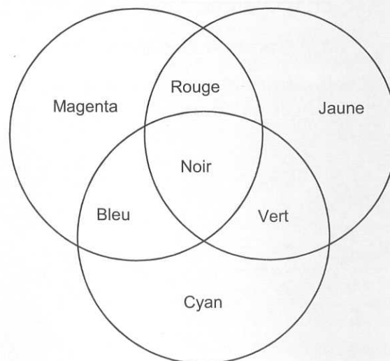
Synthèse soustractive
