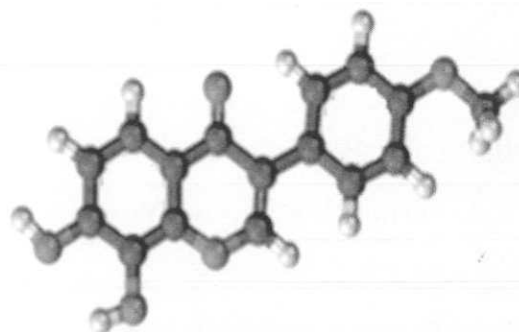
Modélisation d'une molécule d'isoflavone (logiciel Rastop)
