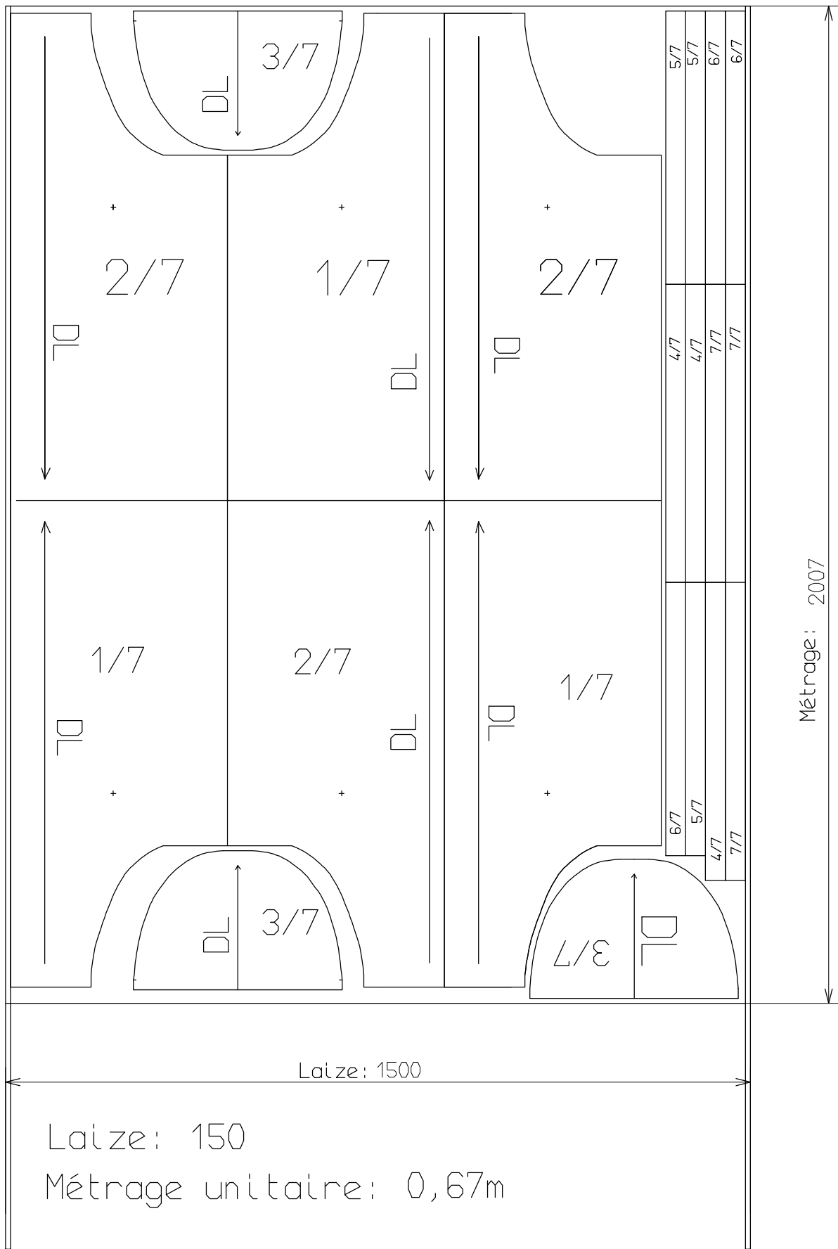
TRACE de REFERENCE DU TABLIER 88-35
