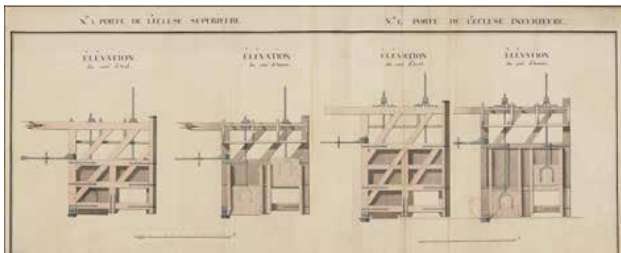
Ecluse en coupe, planche aquarellée, 1773. Arch. dép. Charente 1 C 92
