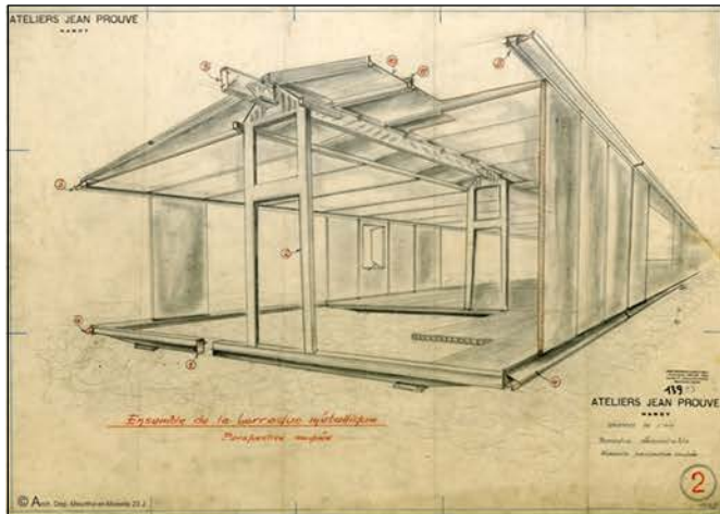
Maison démontable (plan-1939 réalisation 1944)
